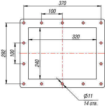
Выходной фланец
