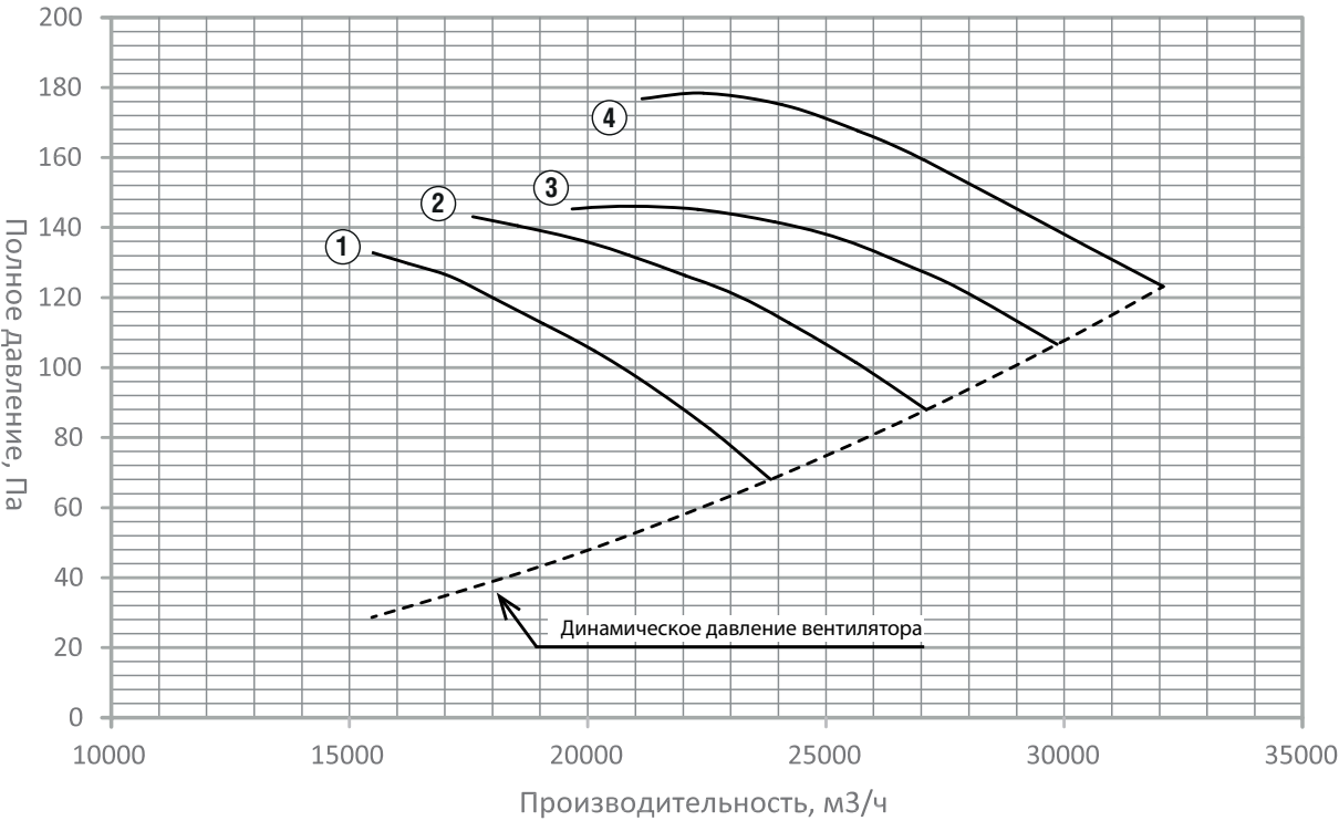
① В0 21-12 №9 9С (1,1/750) ③ В0 21-12 №9 9Х (1,5/750) ② В0 21-12 №9 9Т (1,5/750) ④ В0 21-12 №9 12Х (2,2/750)
