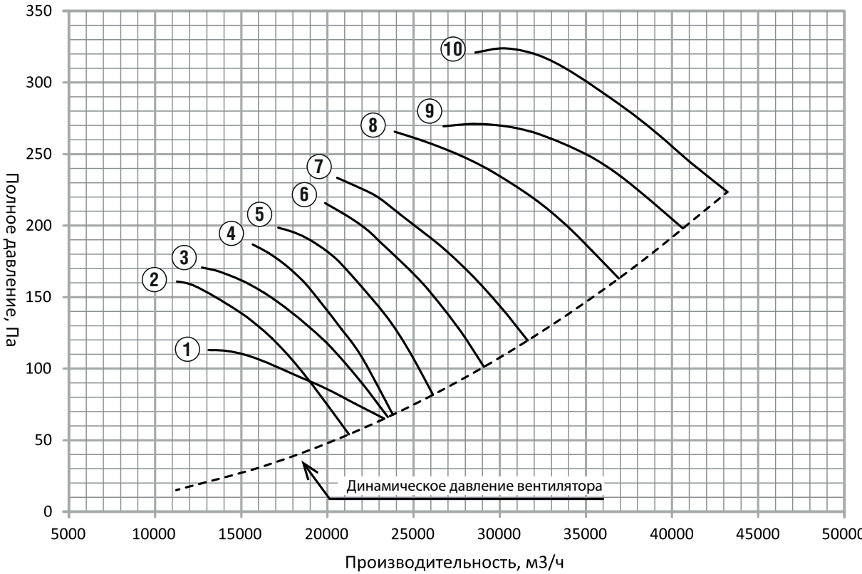
① В0 21-12 №9 3О (0,75/1000) ⑤ В0 21-12 №9 9О (1,5/1000) ⑨ В0 21-12 №9 9Х (4/1000) ② В0 21-12 №9 7М (1,1/1000) ⑥ В0 21-12 №9 9Р (2,2/1000) ⑩ В0 21-12 №912 Х (5,5/1000) ③ В0 21-12 №9 7Н (1,1/1000) ⑦ В0 21-12 №9 9С (2,2/1000) ④ В0 21-12 №9 9Н (1,5/1000) ⑧ В0 21-12 №9 9Т (3/1000)
