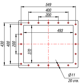
Выходной фланец
