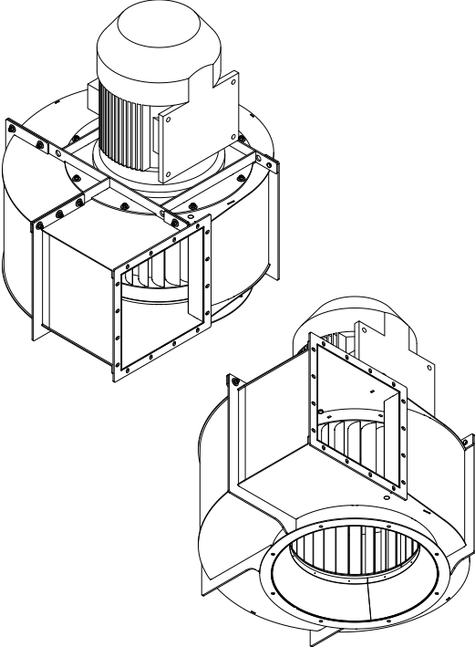
Монтаж на входной фланец
