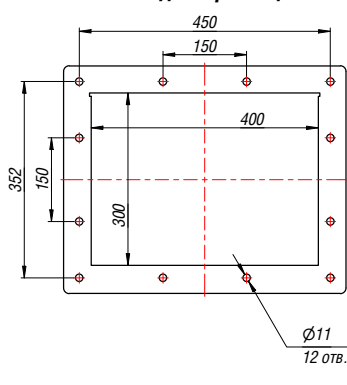
Выходной фланец
