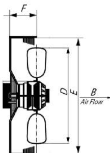
Компактный осевой вентилятор с защитной решеткой и монтажной панелью YWF B
