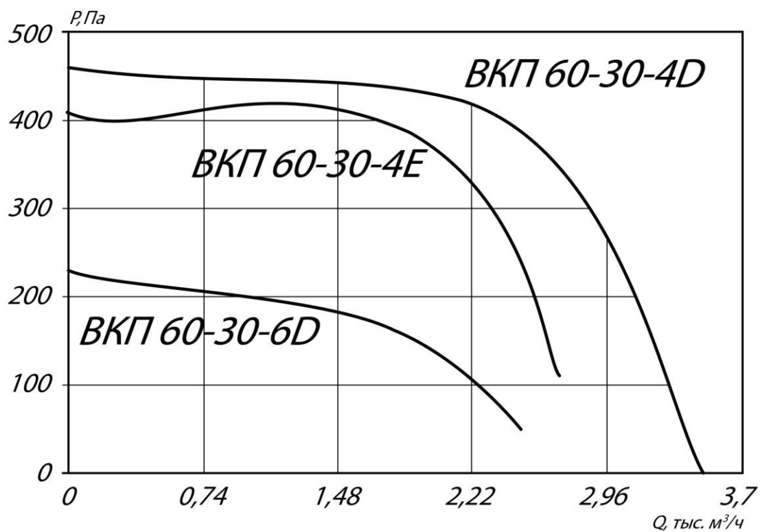
Аэродинамическая характеристика вентилятора ВКП 60-30
