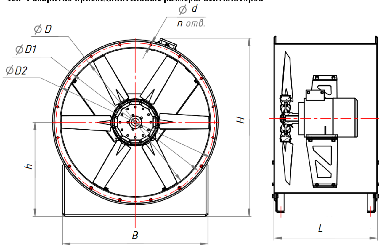
Рисунок 1. Габаритные и присоединительные размеры вентилятора
