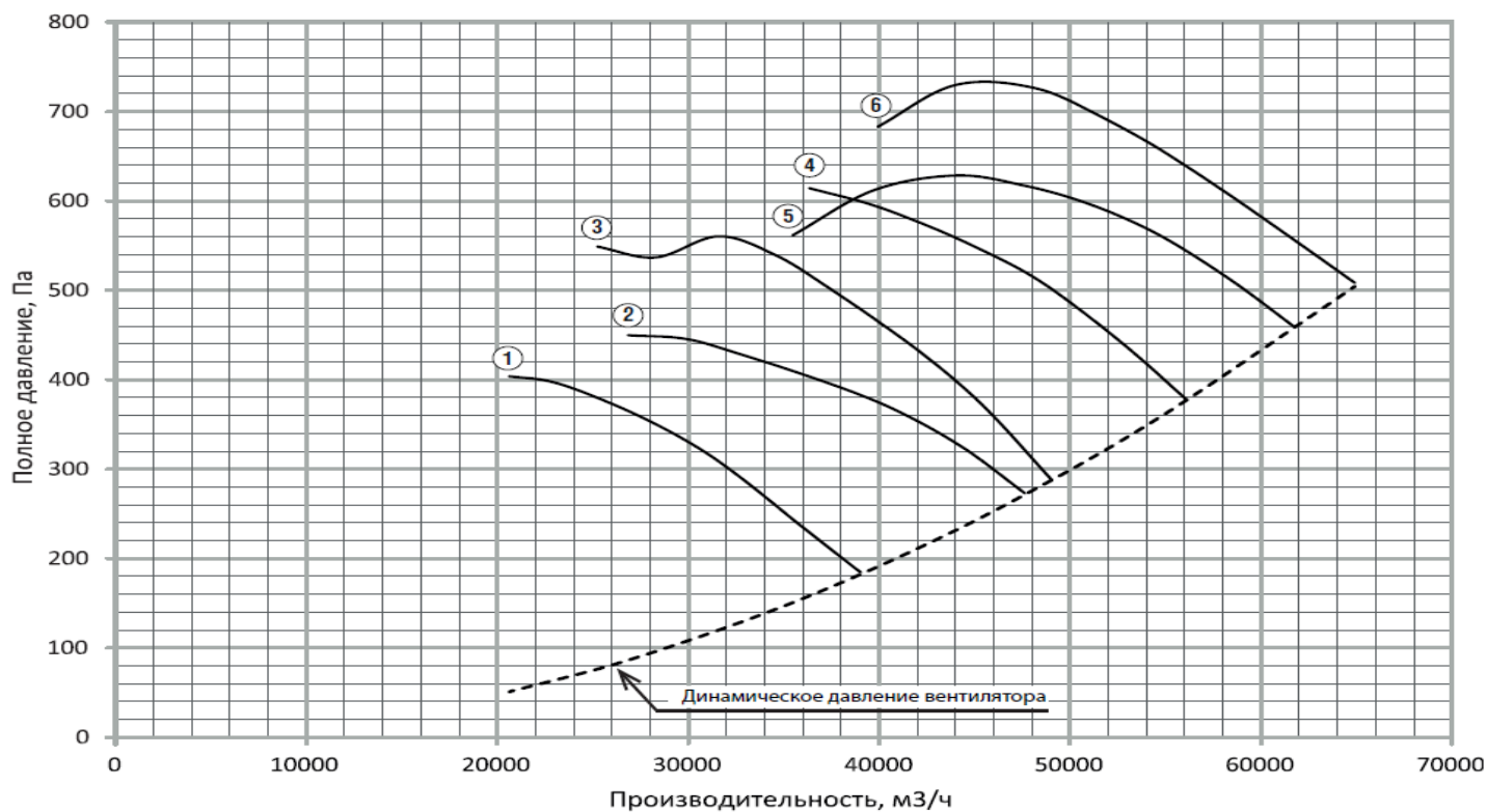
Рисунок 10. Аэродинамическая характеристика вентилятора ВО 21-12 №9 1500 об/мин
