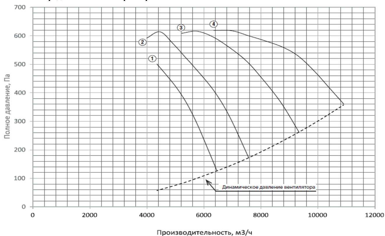
Рисунок 2. Аэродинамическая характеристика вентилятора ВО 21-12 №4
