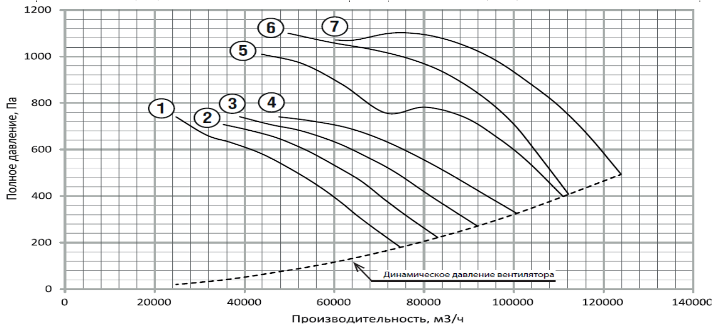
Рис. 13 Аэродинамическая характеристика ВО 21-12 №12,5 1500 об/мин
