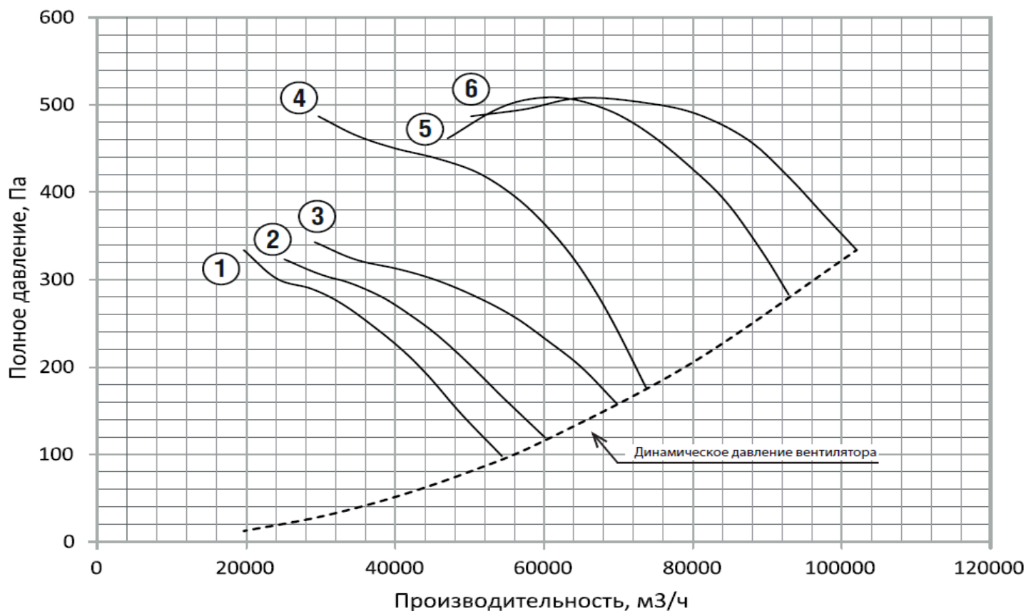
Рис. 12 Аэродинамическая характеристика ВО 21-12 №12,5 1000 об/мин
