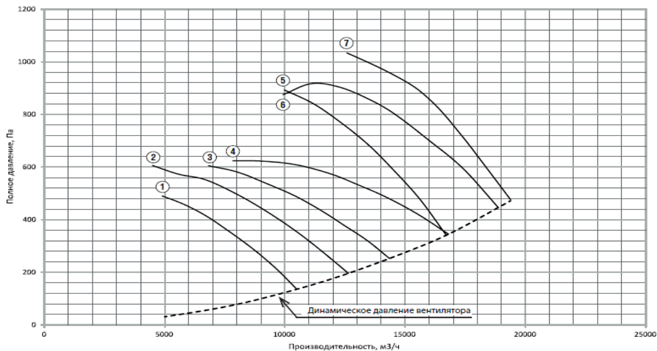
Рисунок 4. Аэродинамическая характеристика вентилятора ВО 21-12 №5
