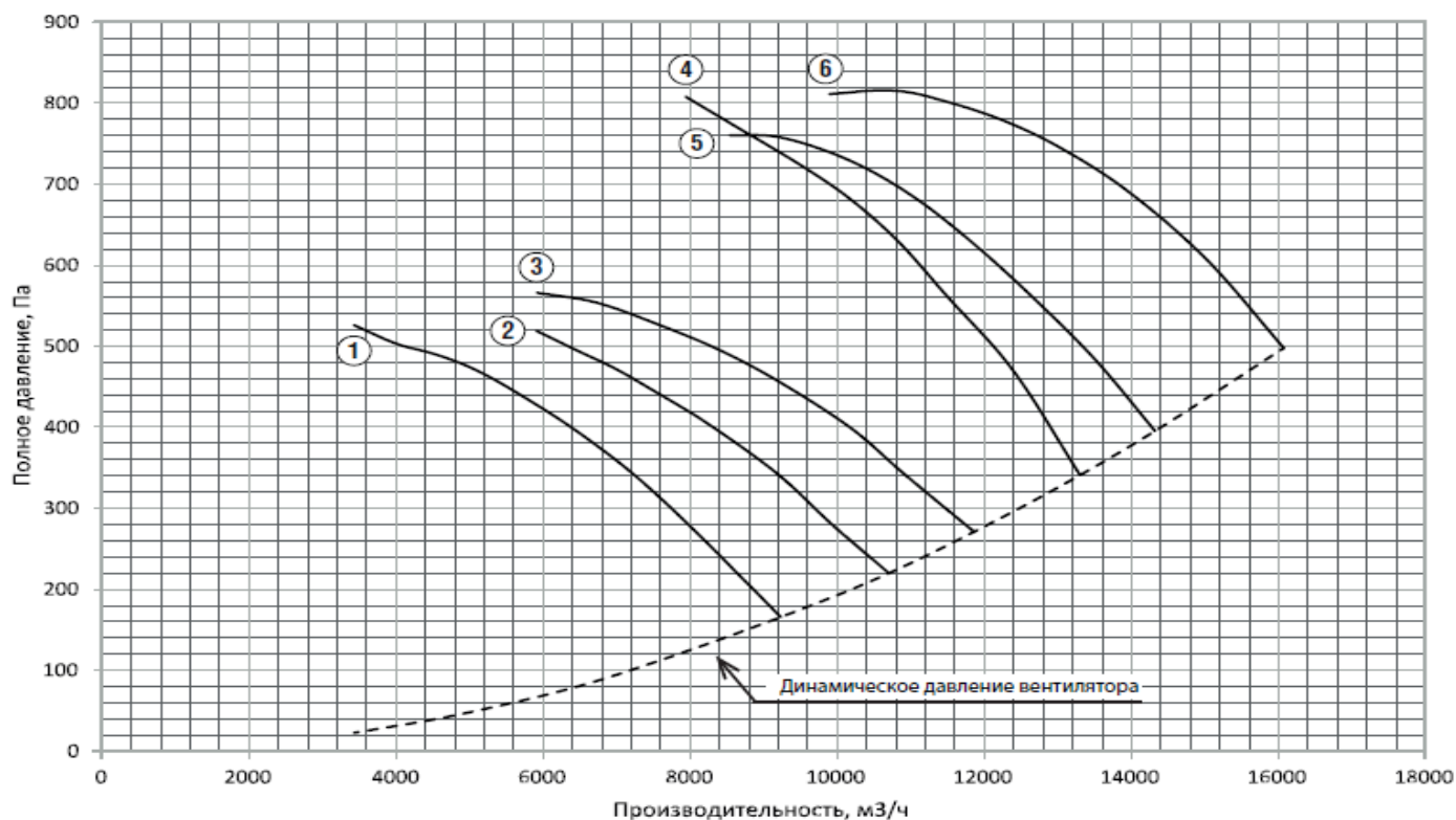
Рисунок 3. Аэродинамическая характеристика вентилятора ВО 21-12 №4,5
