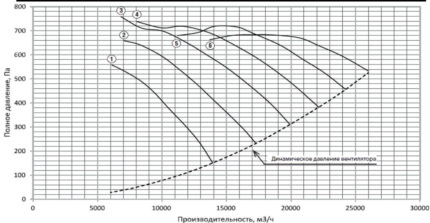
Рисунок 5. Аэродинамическая характеристика вентилятора ВО 21-12 №5,6
