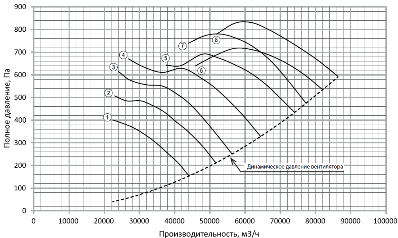
Рисунок 11. Аэродинамическая характеристика вентилятора ВО 21-12 №10 1500 об/мин
