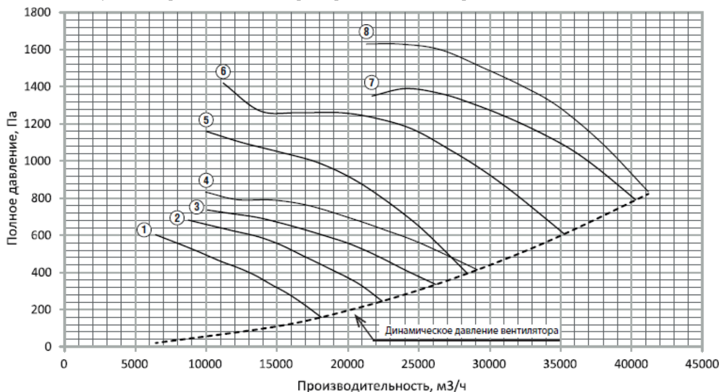
Рисунок 6. Аэродинамическая характеристика вентилятора ВО 21-12 №6,3
