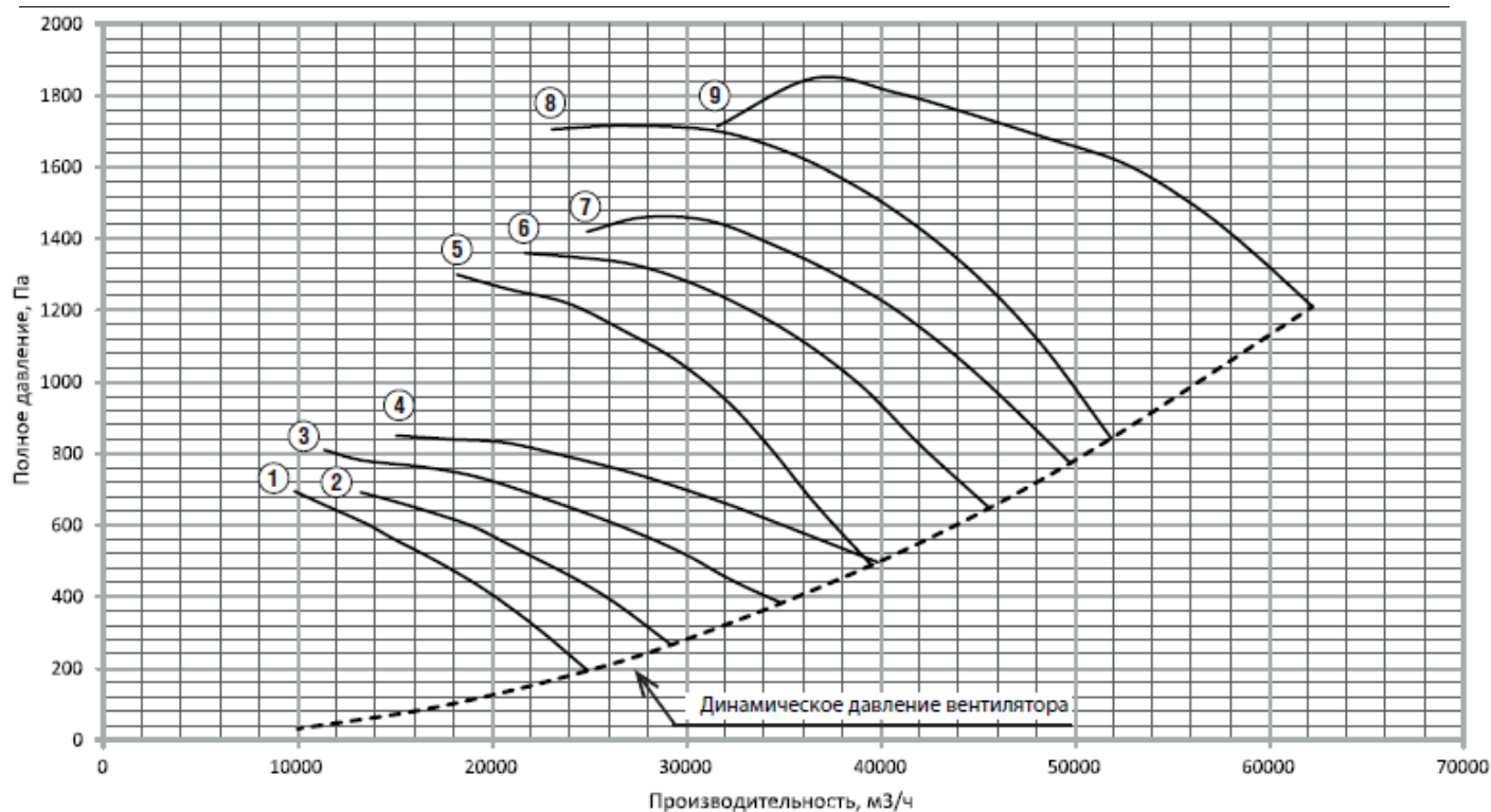
Рисунок 7. Аэродинамическая характеристика вентилятора ВО 21-12 №7,1
