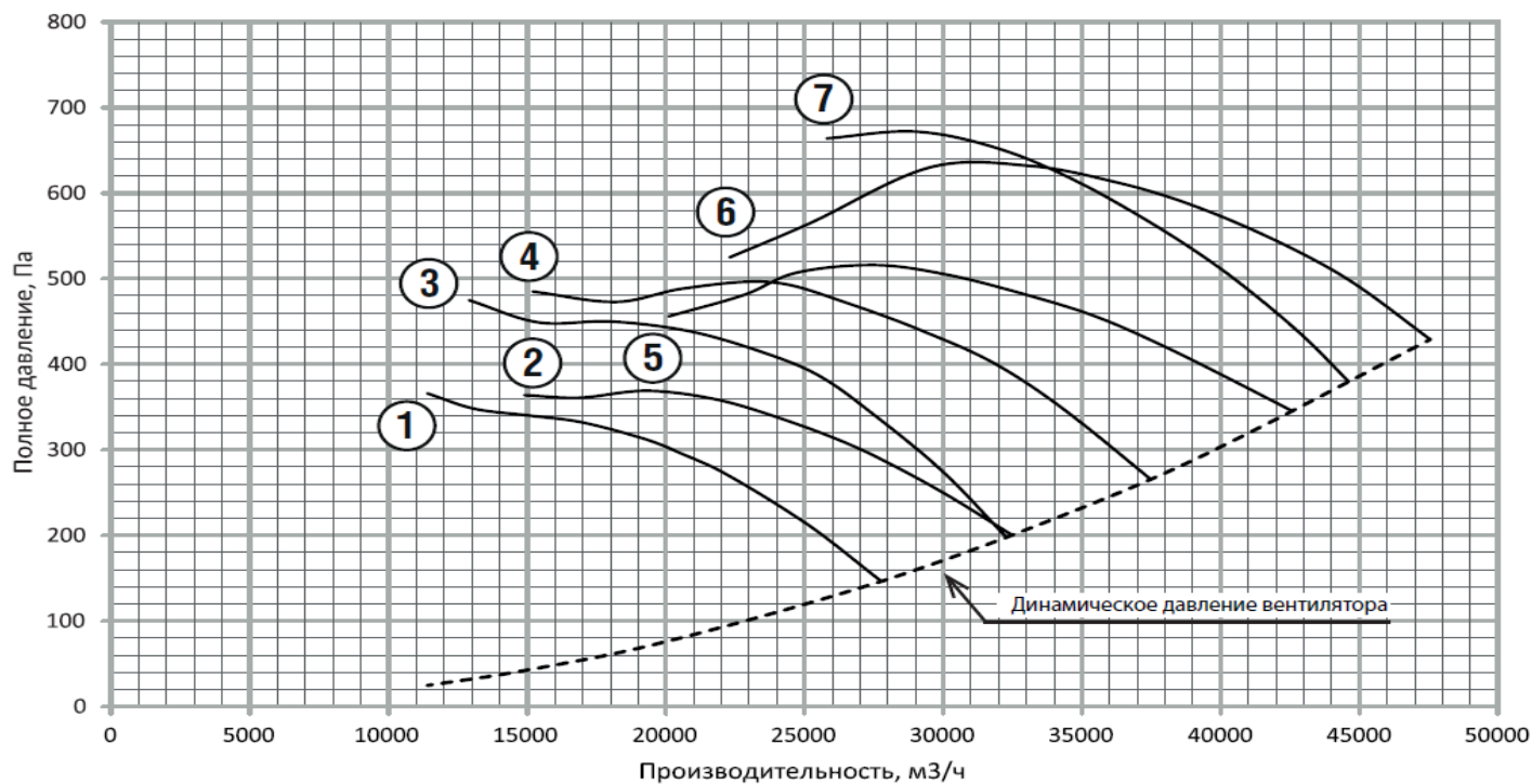
Рисунок 8. Аэродинамическая характеристика вентилятора ВО 21-12 №8 1500 об/мин
