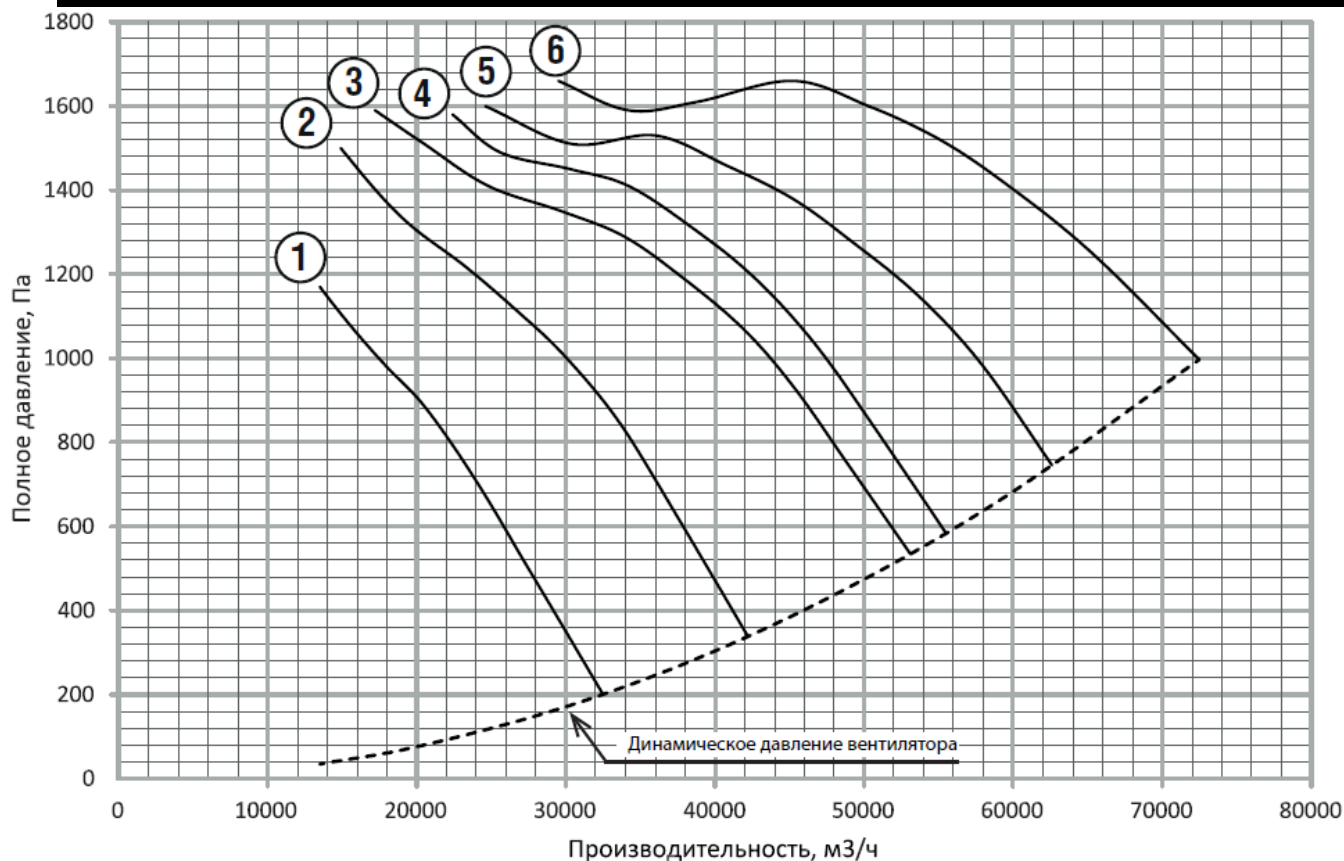
Рисунок 9. Аэродинамическая характеристика вентилятора ВО 21-12 №8 3000 об/мин
