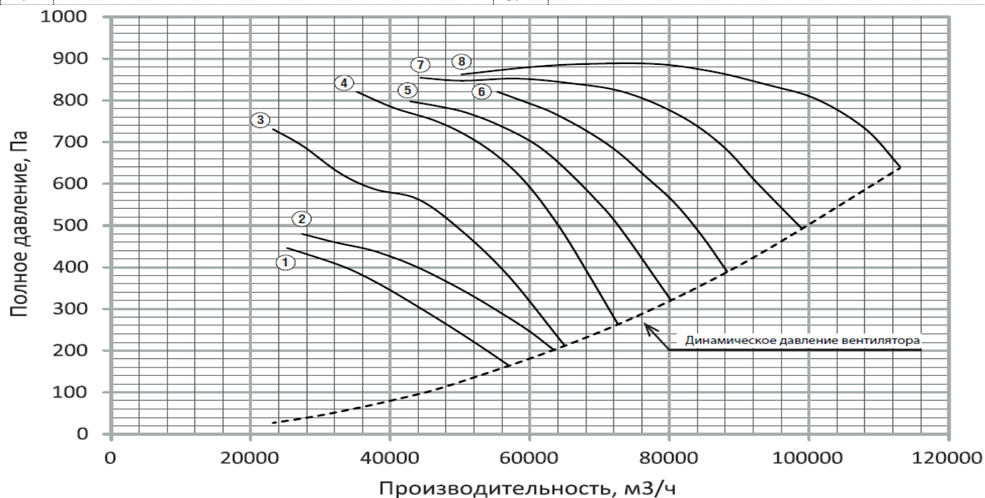
Рис 12. Аэродинамическая характеристика вентилятора ВО 21-12 №11,2 1500 об/мин.
