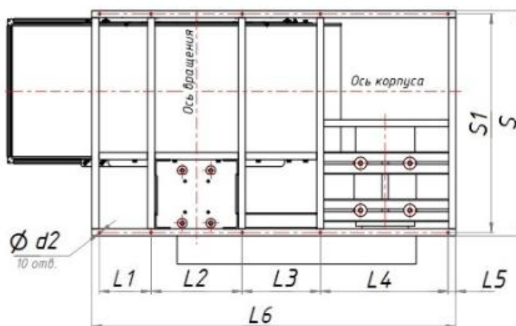
Для ВР 80-75 №10, ВР 80-75 №12,5 исполнение 5
