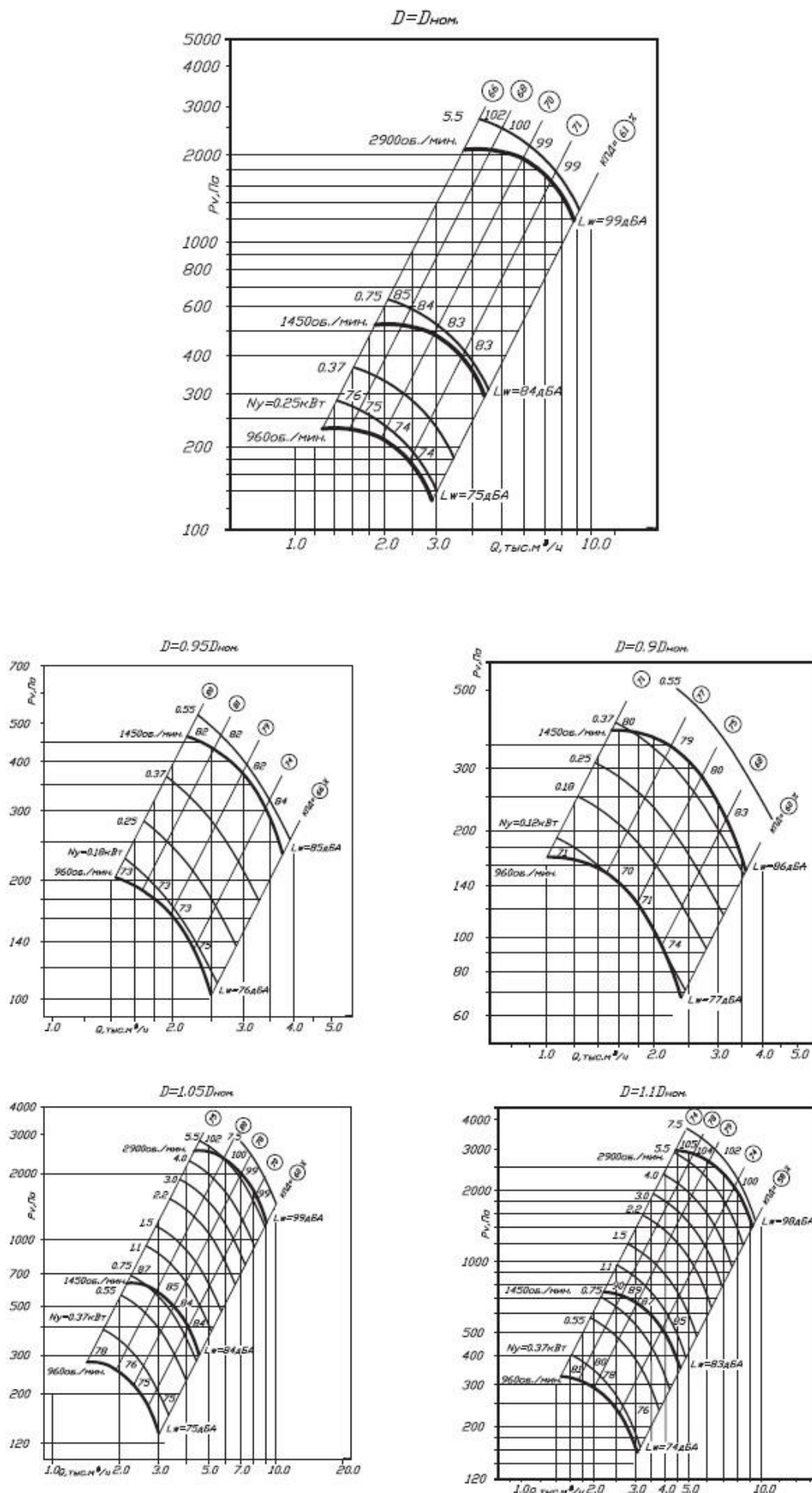
Аэродинамическая характеристика вентилятора ВР 80-75 №4 сх.1
