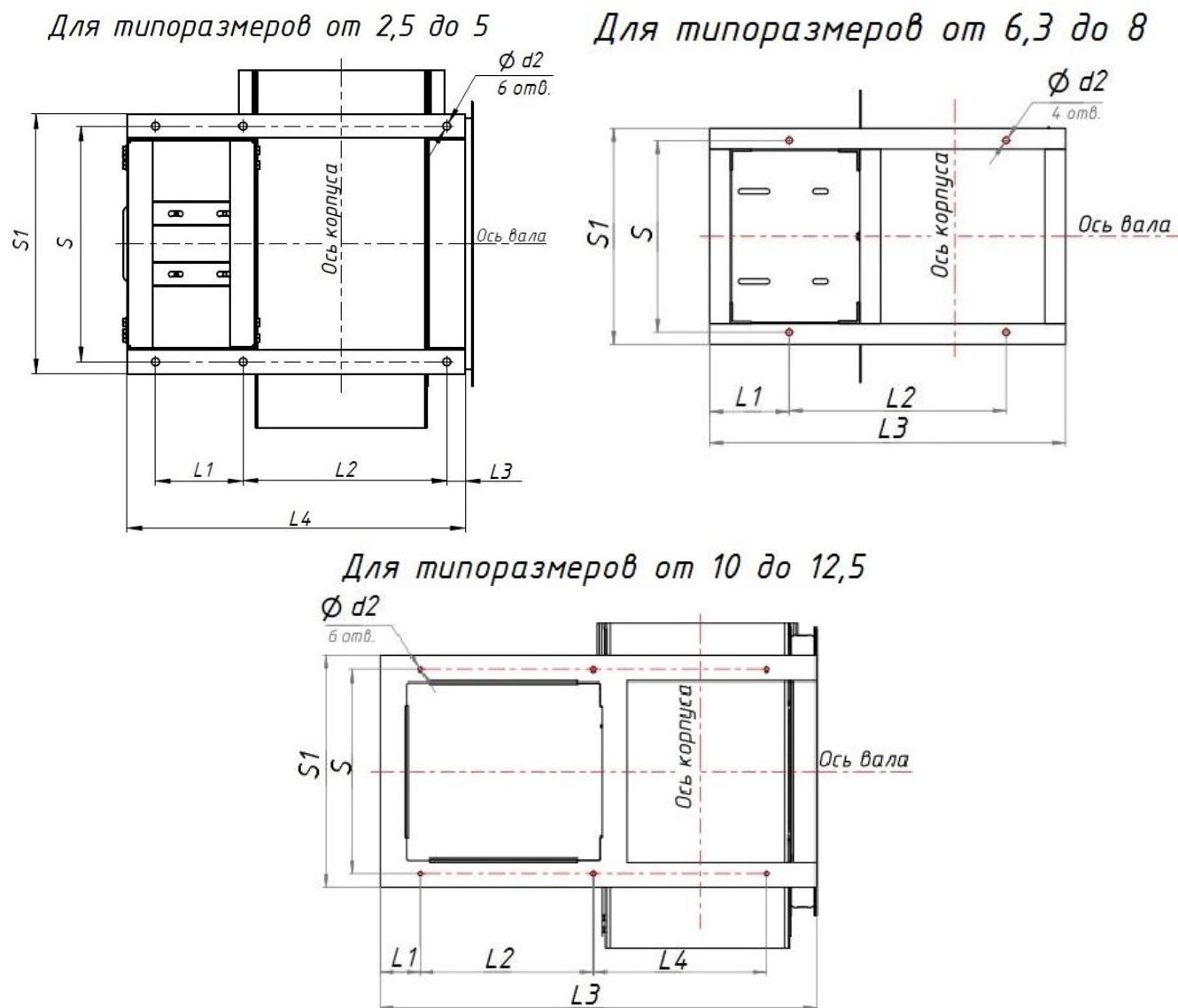
Рисунок 2. Основание рамы вентиляторов ВР 80-75
