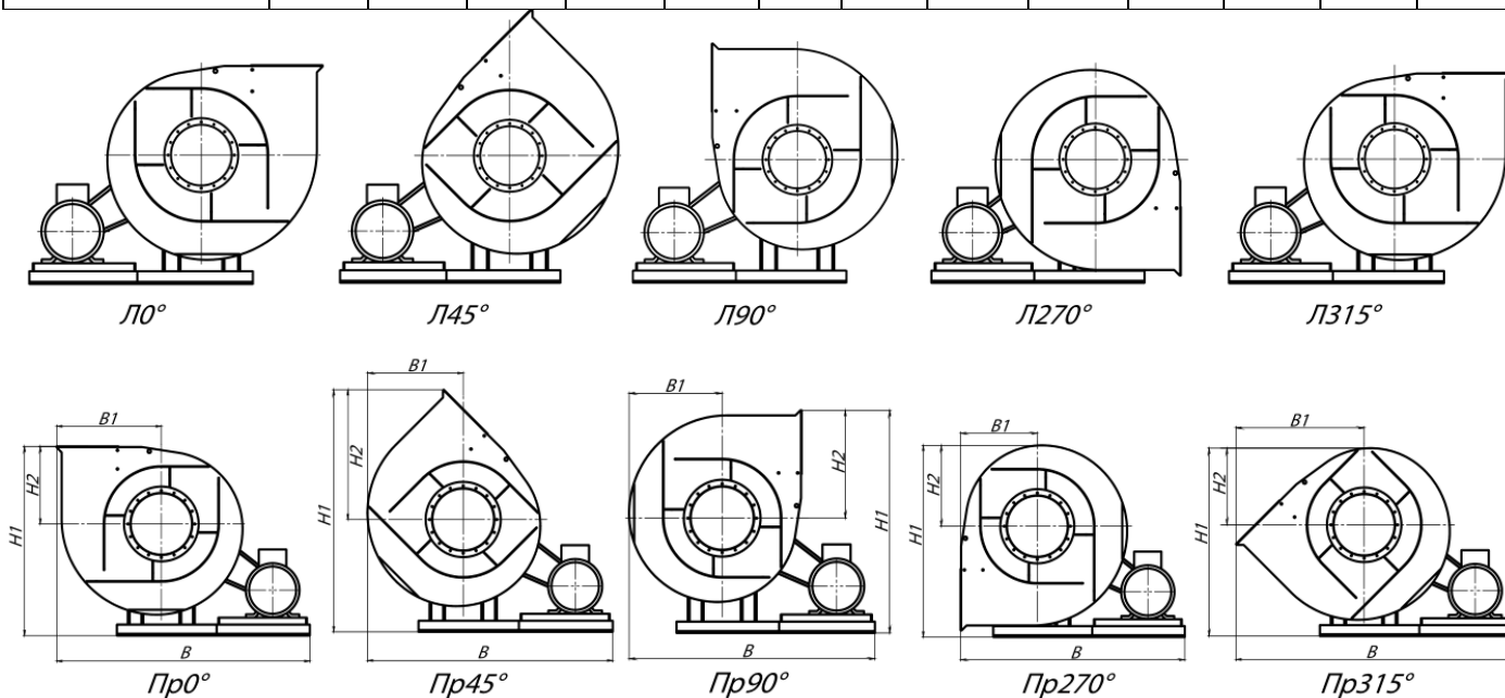
Рисунок 5. Габаритные размеры вентиляторов исполнение 5 в зависимости от положения корпуса
