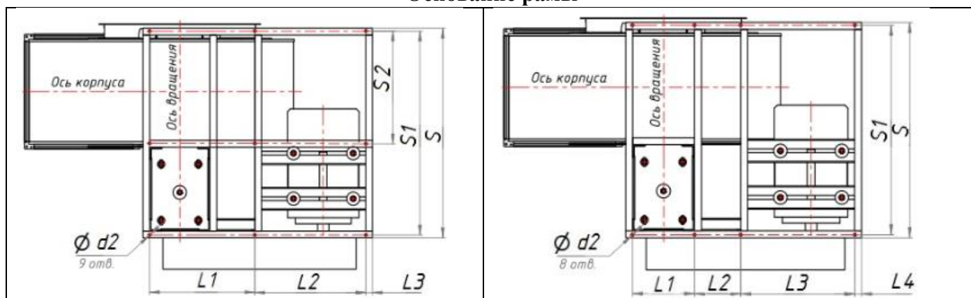
Для ВР 80-75 №6,3 исполнение 5
