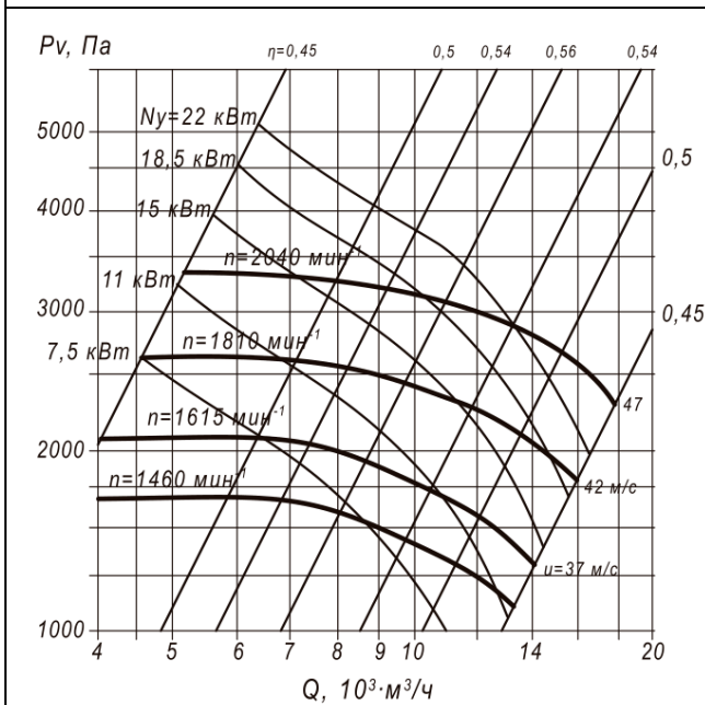
Аэродинамическая характеристика вентилятора ВЦП 7-40 №4
