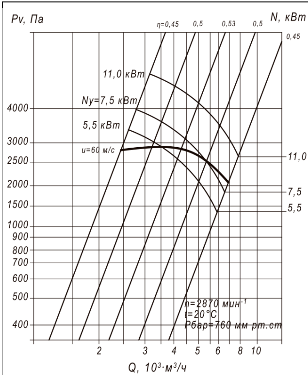
Аэродинамическая характеристика вентилятора ВЦП 7-40 №4
