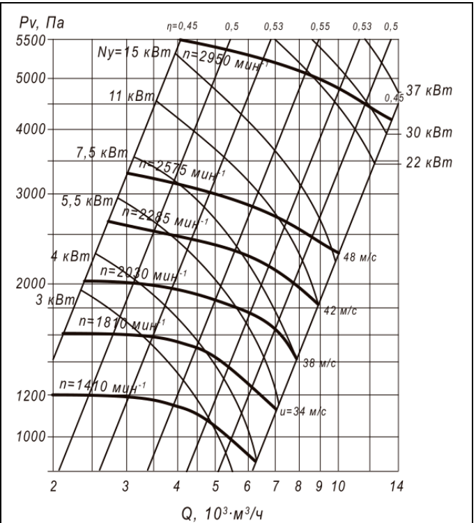
Аэродинамическая характеристика вентилятора ВЦП 7-40 №5
