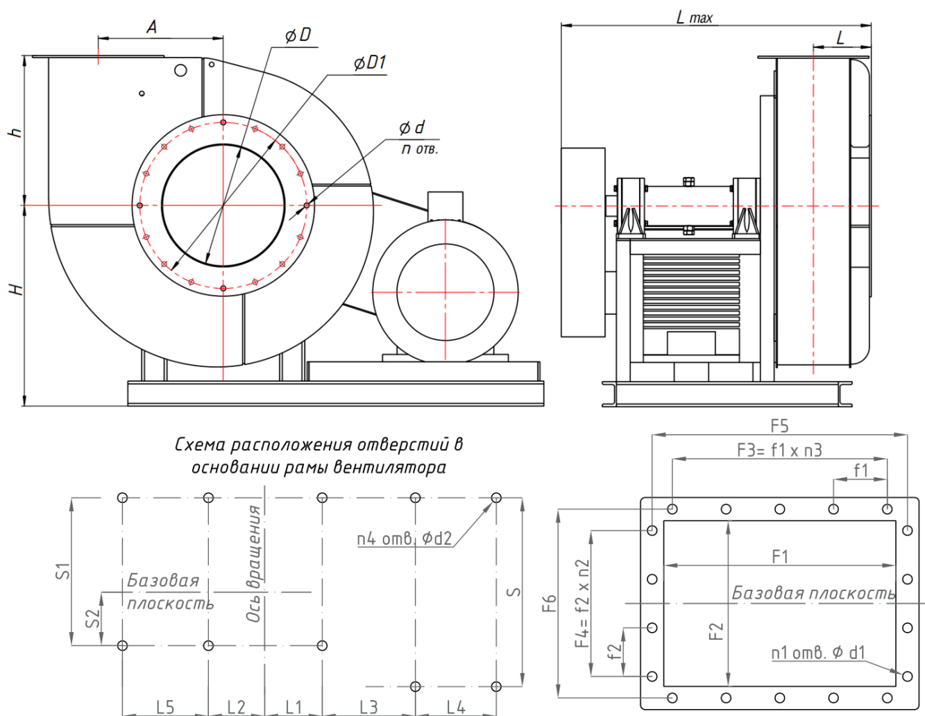
Рисунок 3- габаритные,присоединительные размеры вентиляторов
