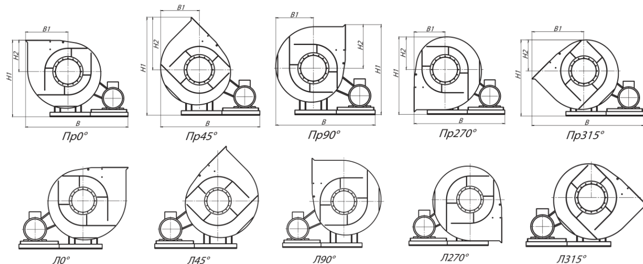
Рисунок 4- габаритные размеры вентиляторов
