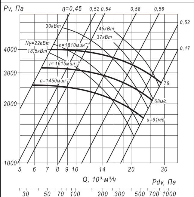
Аэродинамическая характеристика вентилятора ВЦП 7-40 №5
