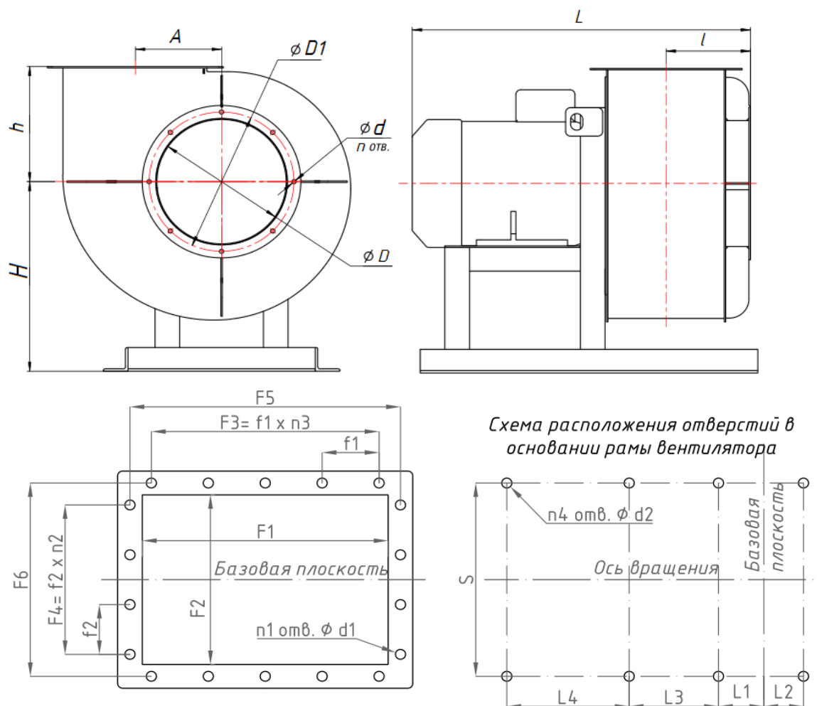
Рисунок 1. Габаритные и присоединительные размеры вентиляторов ВЦП 7-40
