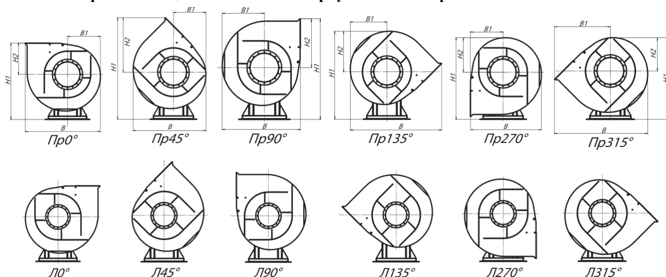
Рисунок 2- размеры зависящие от положения корпуса
