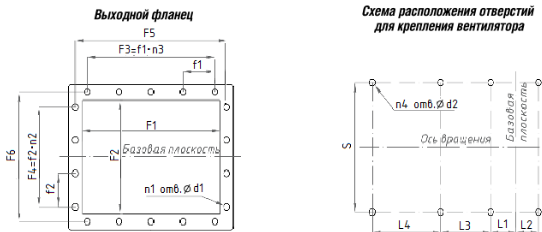
Рис.2. Габаритные и присоединительные размеры вентиляторов ВР 12-26
