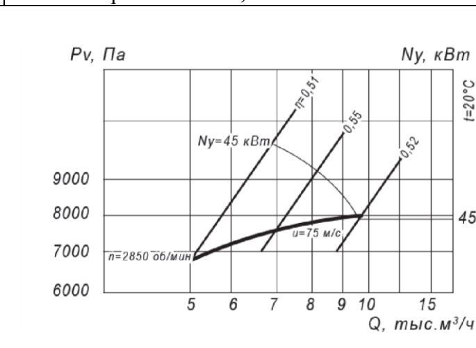
Рис.8.Аэродинамические характеристики вентилятора ВР 12-26-5
