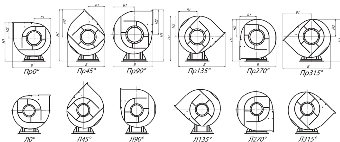
Рис.3. Положение корпуса вентилятора ВР 12-26
