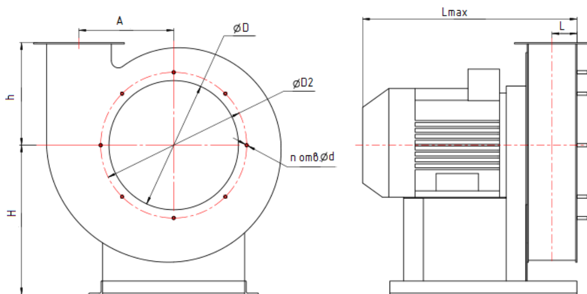
Рис.1. Габаритные и присоединительные размеры вентиляторов ВР 12-26
