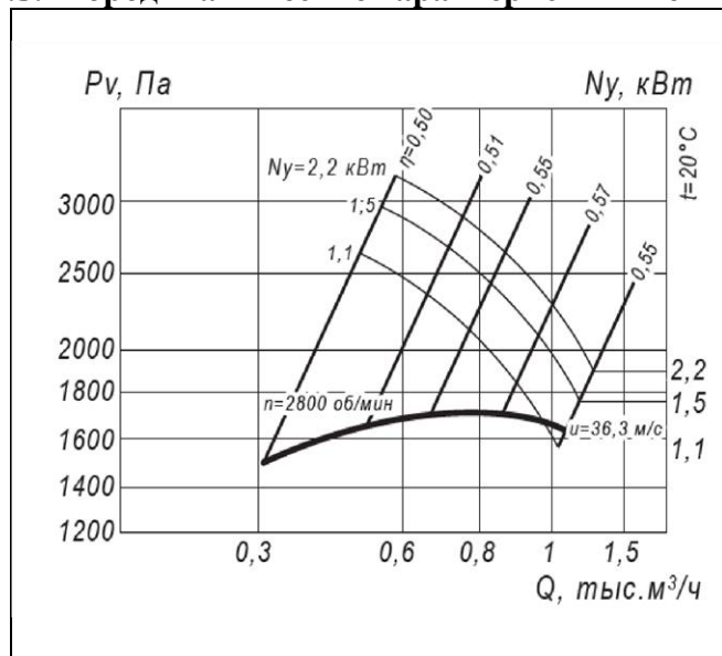
Рис.4.Аэродинамические характеристики вентилятора ВР 12-26-2,5
