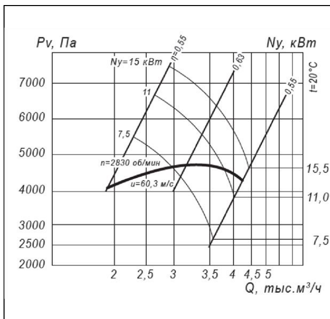
Рис.6.Аэродинамические характеристики вентилятора ВР 12-26-4
