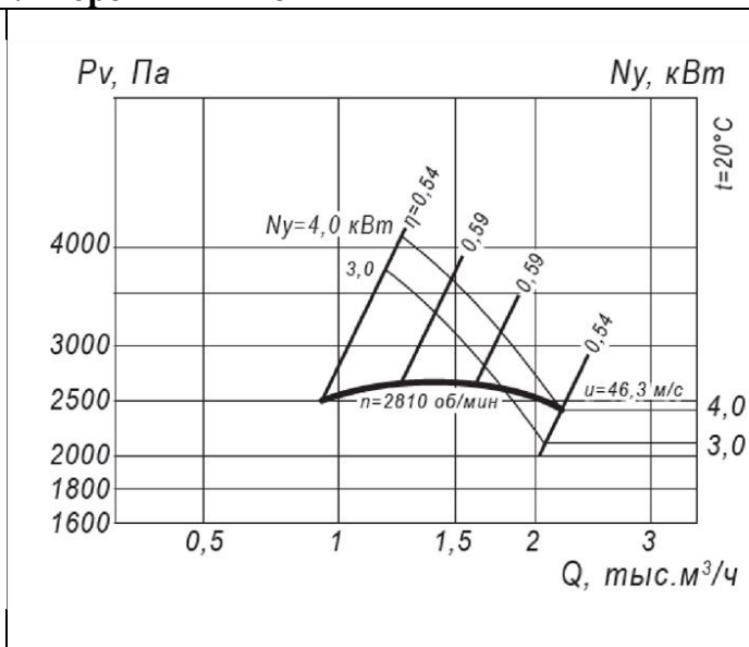
Рис.5.Аэродинамические характеристики вентилятора ВР 12-26-3,15
