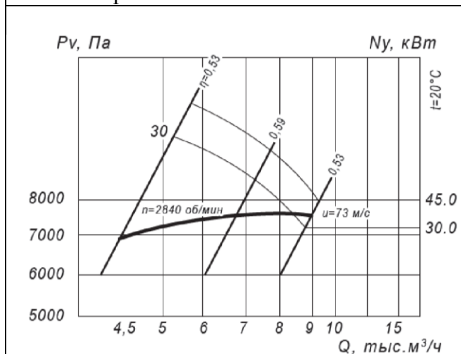
Рис.8.Аэродинамические характеристики вентилятора ВР 12-26-5
