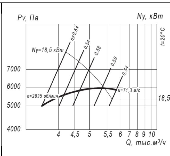
Рис.7.Аэродинамические характеристики вентилятора ВР 12-26-4,5
