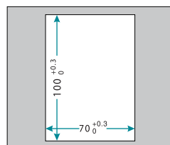
Рисунок 2-13. Размеры пульта без крепежного основания
