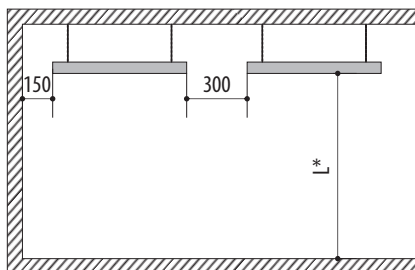
Рисунок 3. Минимальные расстояния от обогревателя до других поверхностей (мм).
